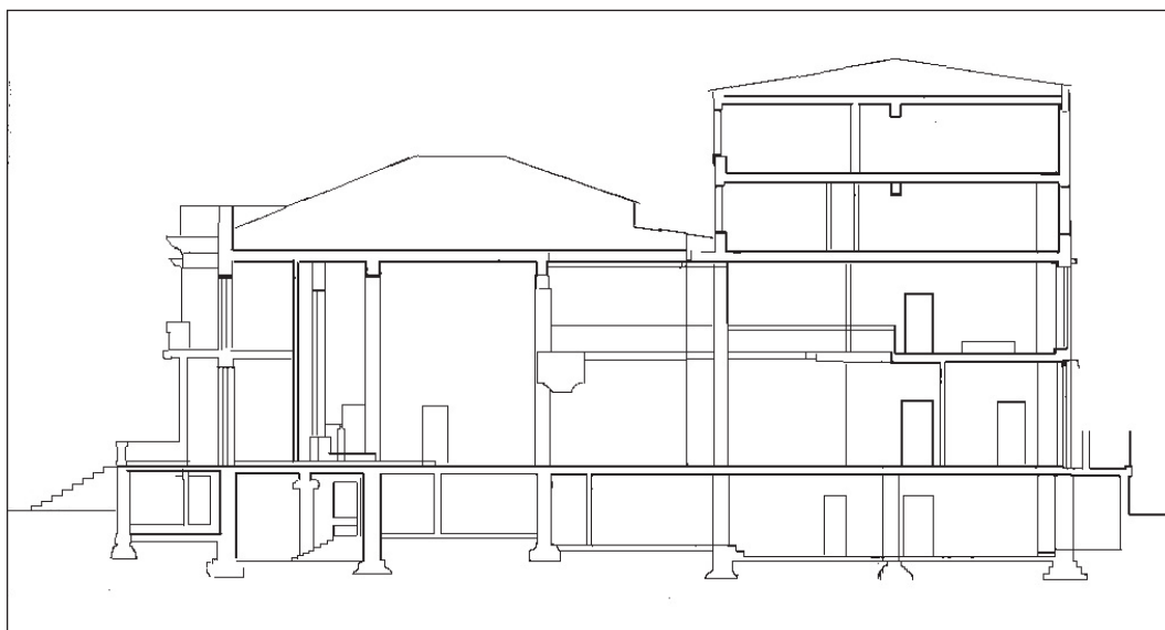
15. Projekt wnętrza kościelnego, uzyskanego w wyniku połączenia z budynkiem planowanym od ul. Narbutta, niezrealizowany. Bez daty. Archiwum Prowincji Wielkopolsko-Mazowieckiej Towarzystwa Jezusowego, Warszawa. Arch. Stanisław Marzyński (?)
