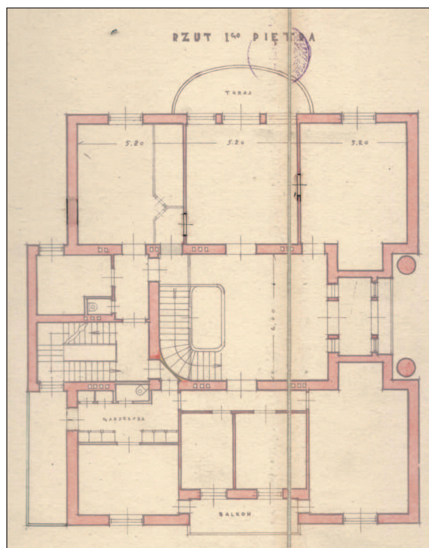
7. Rzut 1 piętra, proj. A. Buraczewski, 1928. Archiwum Prowincji Wielkopolsko-Mazowieckiej Towarzystwa Jezusowego, Warszawa, sygn. WaN 3
