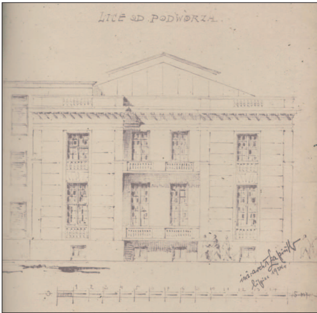
5. Elewacja południowa, proj. T. Łapiński, 1924. Archiwum Prowincji Wielkopolsko-Mazowieckiej Towarzystwa Jezusowego, Warszawa, sygn. WaN 2.
