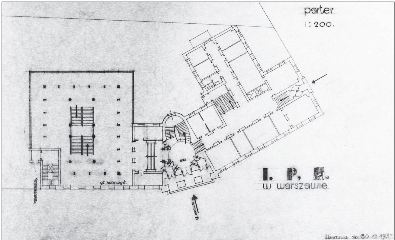
4. Z. Mączyński, projekt koncepcyjny pierwszej rozbudowy gmachu Izby Przemysłowo – Handlowej w Warszawie przy ul. Senackiej, róg Wiejskiej – rzut parteru. Rys. datowany: 30.XII.1937. Archiwum domowe rodziny architekta
